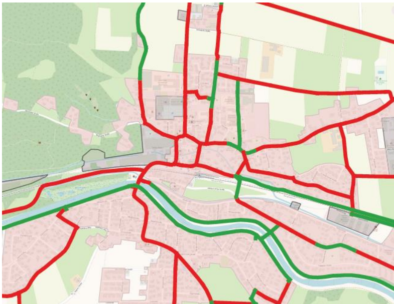
Abbildung 14: Netzkarte mit Hervorhebung der Netzlücken/ungesicherter Abschnitte (rot)
